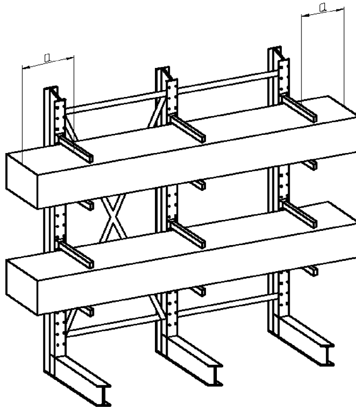
Рисунок 11. Размещение грузов на консольных стеллажах
